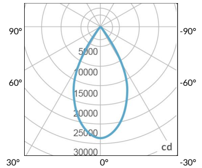
Beam Angle : 50°
